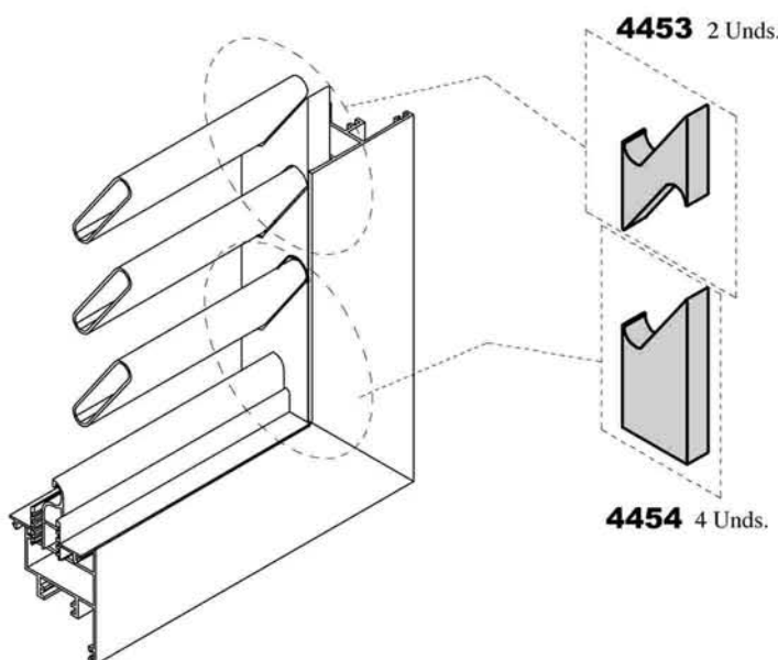
ESQUEMA DE COLOCACION DE POSICIONAMIENTO CELOSIA FIJA ,CON PERFIL DE LAMA FIJA (Ref.: 8309)
